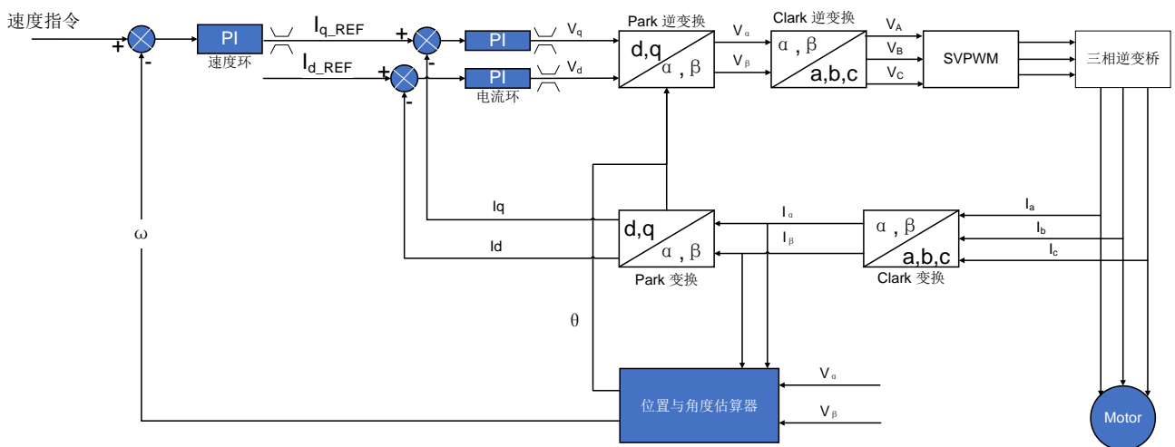
矢量控制应用框图
