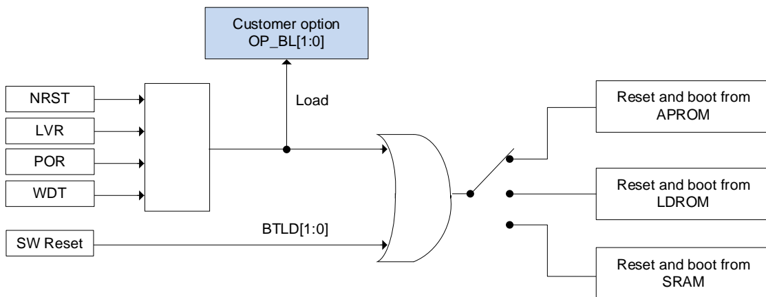
SC32M15X 复位后启动区域切换示意图
