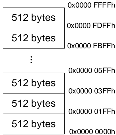
SC32M15X 系列 64 Kbytes APROM Sector 分区示意
