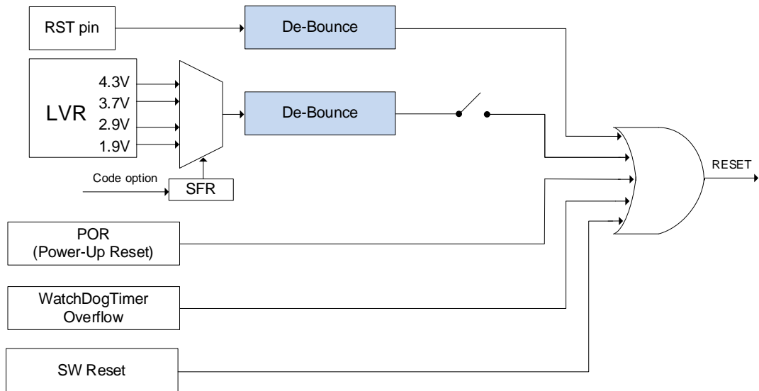
SC32M15X 复位电路图
